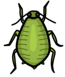
aphids
